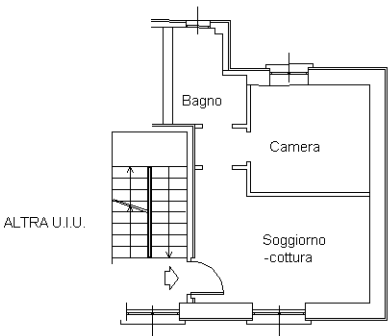
Pianta Piano Primo h=mt.2.70
