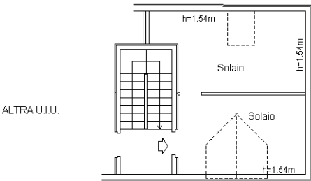
Pianta Piano Terzo
