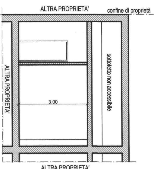
SEZIONE A-A
