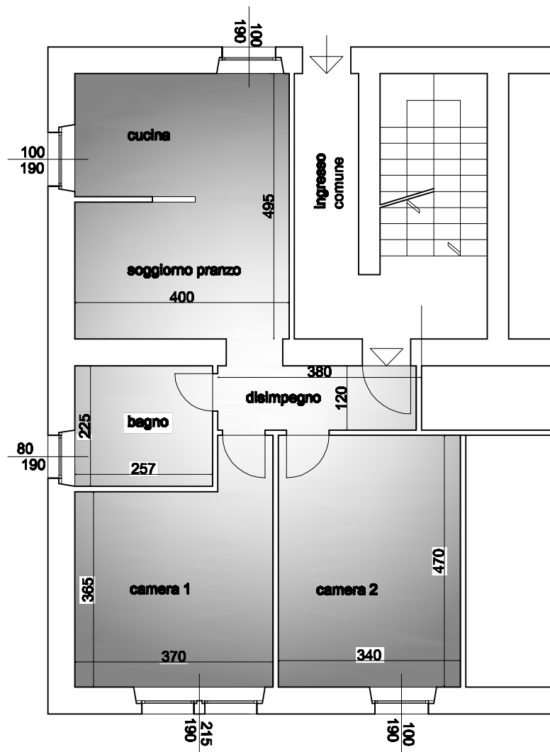
PLANIMETRIA scala 1:100
