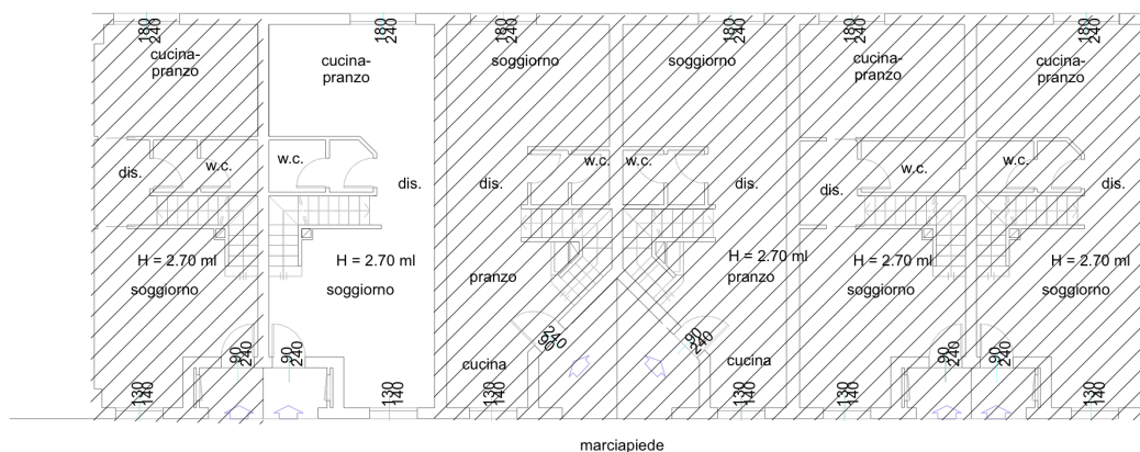
PIANTA PIANO TERRENO - Rapp. 1:200
