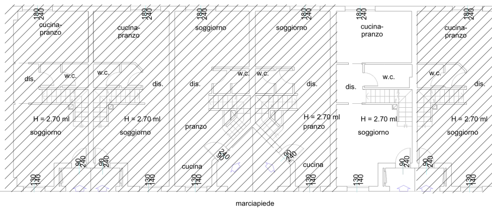
PIANTA PIANO TERRENO - Rapp. 1:200
