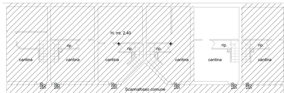
PIANTA PIANO INTERRATO - Rapp. 1:200
