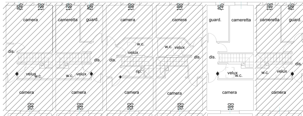
PIANTA PRIMO PIANO - Rapp. 1:200
