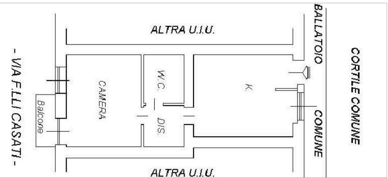
PLANIMETRIA SCALA 1:100 CATASTALE IN ATTI
