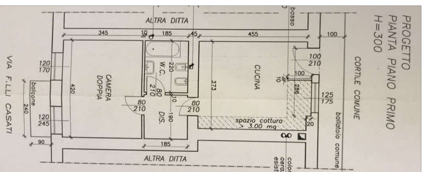
PLANIMETRIA SCALA 1:100 PROGETTO D.I.A. del 09-05-2006
